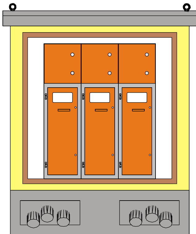
Złącze kablowe rozmieszczenie rozdzielnic wewnątrz
